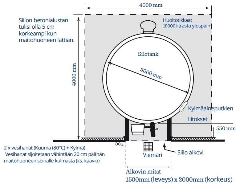
Mueller® Siilon mitat, ylhäältä:
