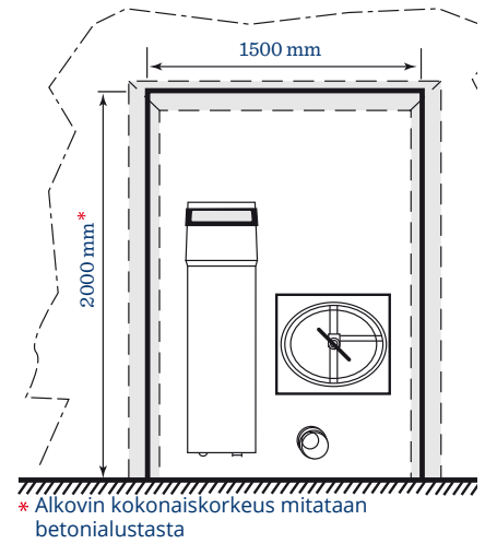
Mueller siilo alkovin mitat, edestä:
