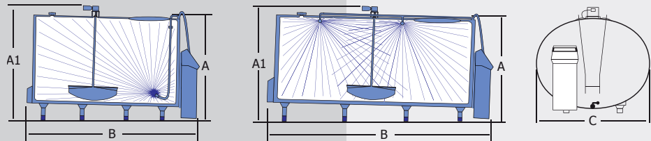
Mallista O-2000 ja P-8000 alkaen säiliöt varustettu suihkusuuttimilla (irroitettava suutinputki).
